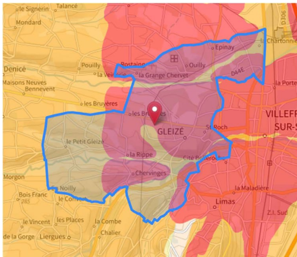
Carte de l'aléa retrait et gonflement des argiles (Source : géorisques.fr).
